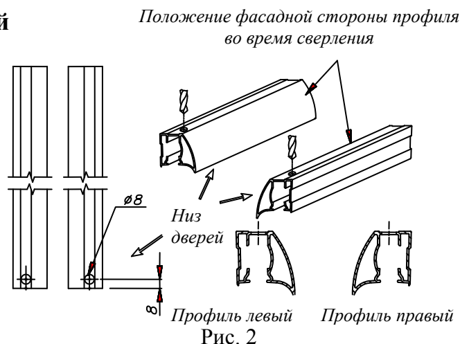
Сверление отверстий в вертикальных профилях
