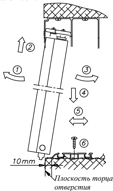
Рис. 10 Установка дверей
