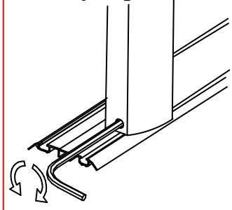
Рис. 14 Регулировка дверей
